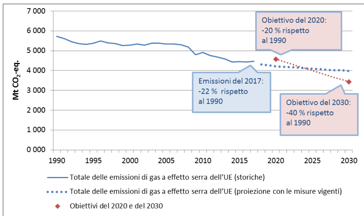
Figura 1: totale delle emissioni di gas a effetto serra (emissioni storiche 1990-2017, proiezione delle emissioni per il 2018-2030) (Mt CO 2 -eq.) e obiettivi di riduzione delle emissioni di gas a effetto serra 1 .
