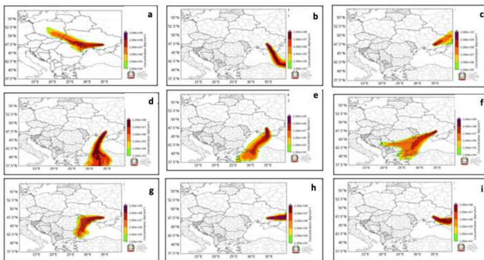
Figura 3: esempi dei risultati ottenuti dalle simulazioni giornaliere effettuate ipotizzando un incidente presso la centrale nucleare ucraina di Zaporizhzhya. Le immagini rappresentano la dispersione dopo 24 ore da un ipotetico rilascio di radioattività in diverse giornate con inizio in data a) 28/8/2022 ore 10, b) 12/2/2023 ore 18 c) 31/12/2022 ore 10 d) 7/2/2023 ore 10 e) 17/3/2023 ore 10 f) 28/5/2023 ore 10 g) 18/4/2023 ore 10 h) 25/9/2022 ore 12 i) 27/12/2022 ore 22
