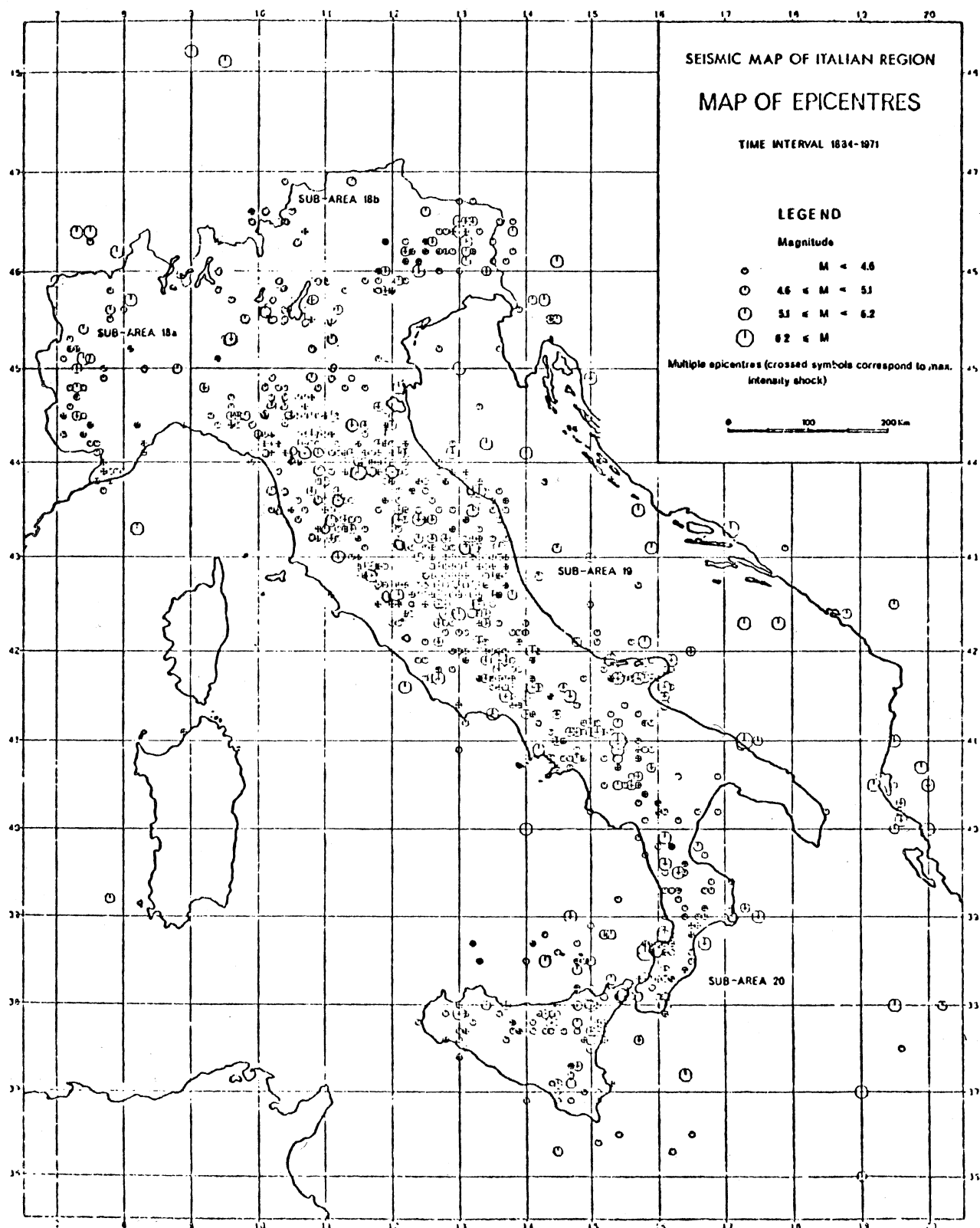
Episcentri, espressi in magnitudo, dei terremoti avvenuti in Italia dal 1884 al 1971 (da Carrozzo, de Visentini, Giorgetti e Springer, 1971).
